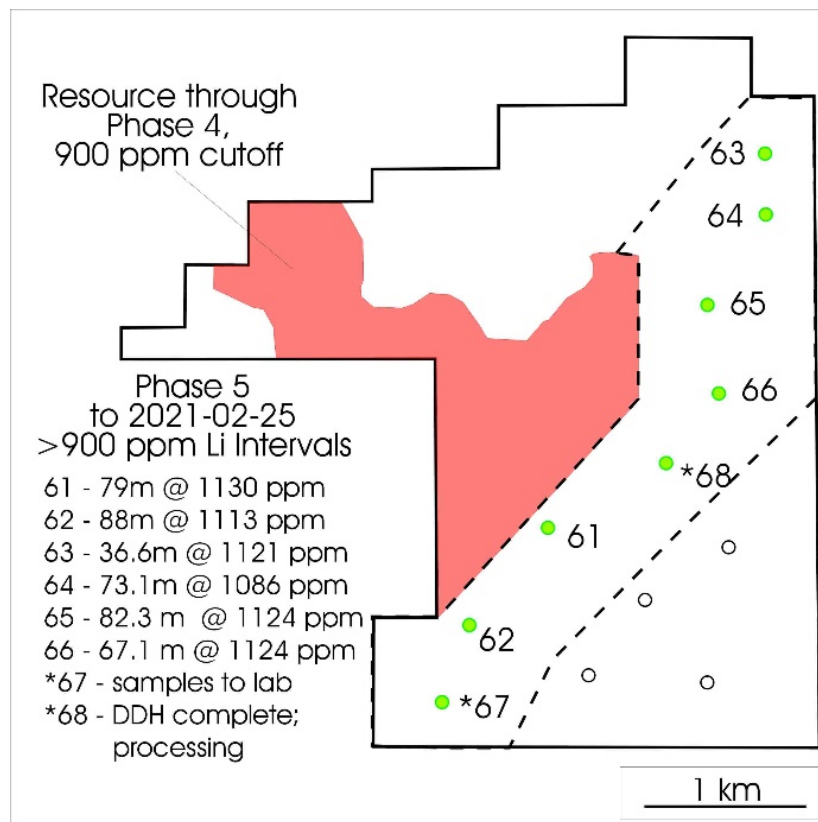
Abbildung 1. Lithium-Ton-Lagerstätte Zeus, 23.3.2021. Die aktuellen angezeigten und abgeleiteten Ressourcen bei einem Cutoff-Gehalt von >900 ppm sind in rot dargestellt und die Lagen der Bohrlöcher der Phase 5 bis Bohrloch CVZ-68 werden gezeigt. Die gestrichelte Linie ist ein hypothetisches Gebiet, das von den Bohrungen der Phase 5 bis heute abgedeckt ist. Die Bohrabstände ähneln denen, die für die Ton-Ressourcen in der Formation Esmeralda in Clayton Valley und in der Nähe verwendet wurden.
